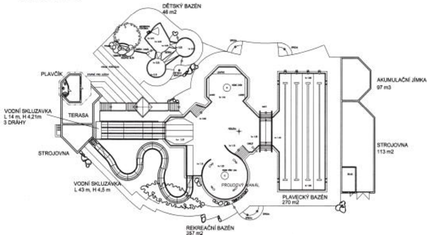
DISPOZICE BAZÉNŮ
